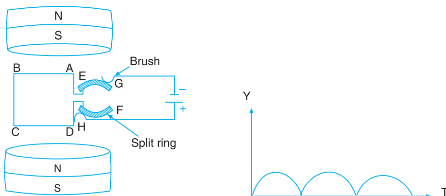
Fig. 17.15 D.C. Generator
